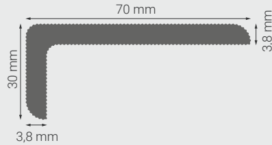
Oberfläche Stark R13
